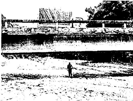
Foto 3. Baja Capacidad Hidráulica.
