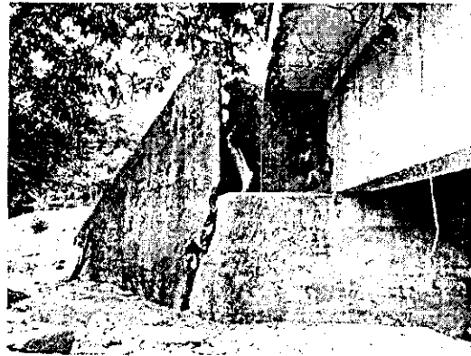
Foto 4. Afectación Estribo- Cost. derecho aguas abajo.
