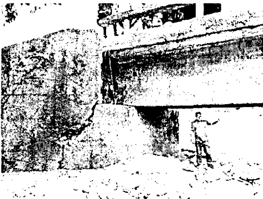
Foto 5. Baja Capacidad Hidráulica y afectación estribo.
